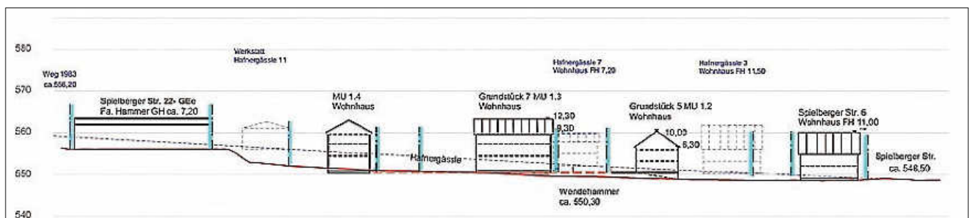
Geländeschnitt West - Ost
